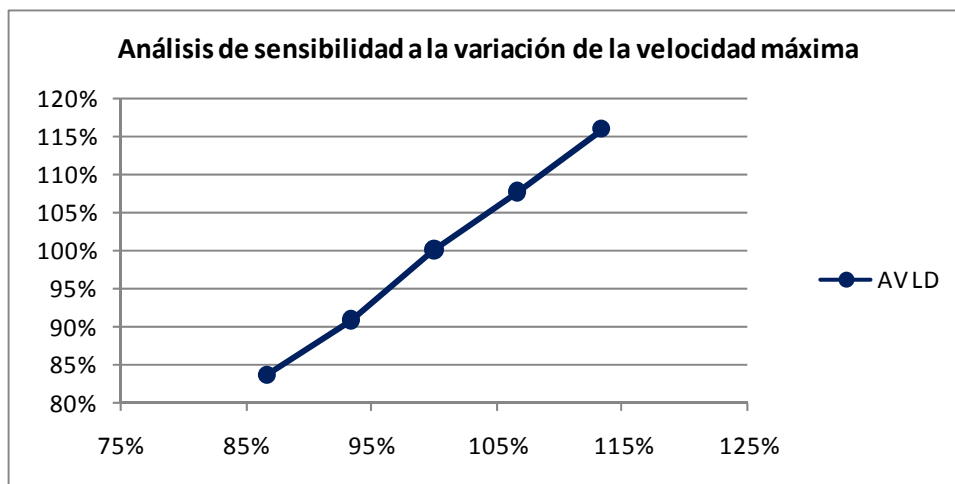
Figura 39. Sensibilidad a la variación de la velocidad máxima
