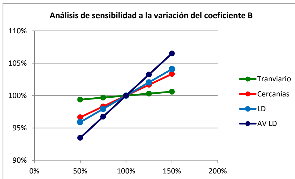
Figura 37. Sensibilidad a la variación del coeficiente B
