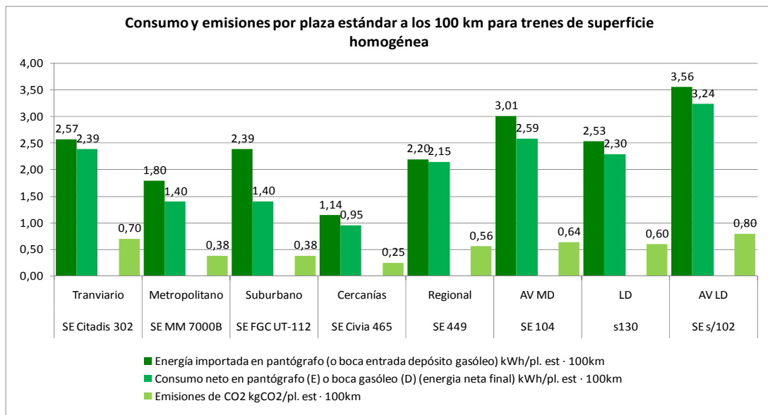
Figura 32. Consumo y emisiones por plaza estándar y kilómetro
