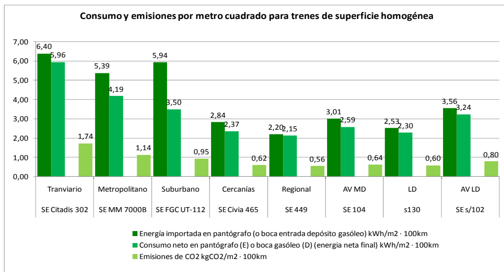
Figura 33. Consumo y emisiones por unidad de superficie y kilómetro
