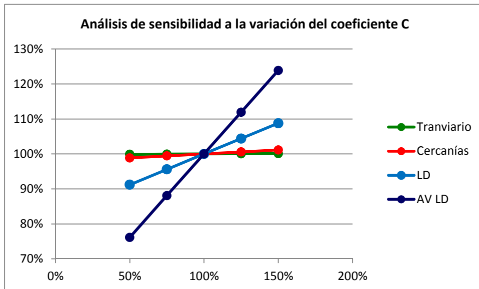
Figura 38. Sensibilidad a la variación del coeficiente C
