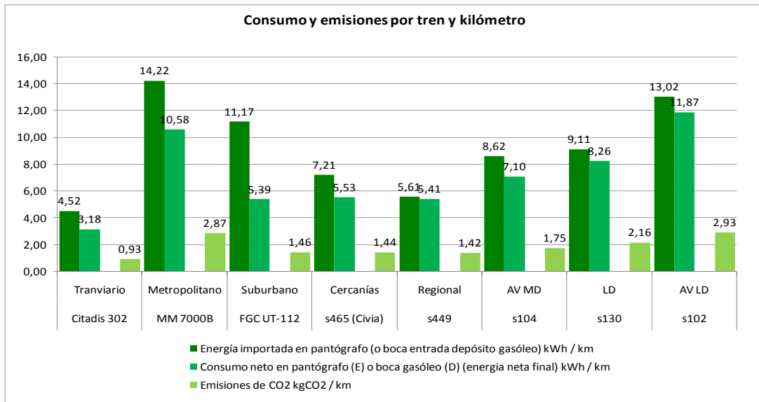
Figura 30. Consumo y emisiones por kilómetro
