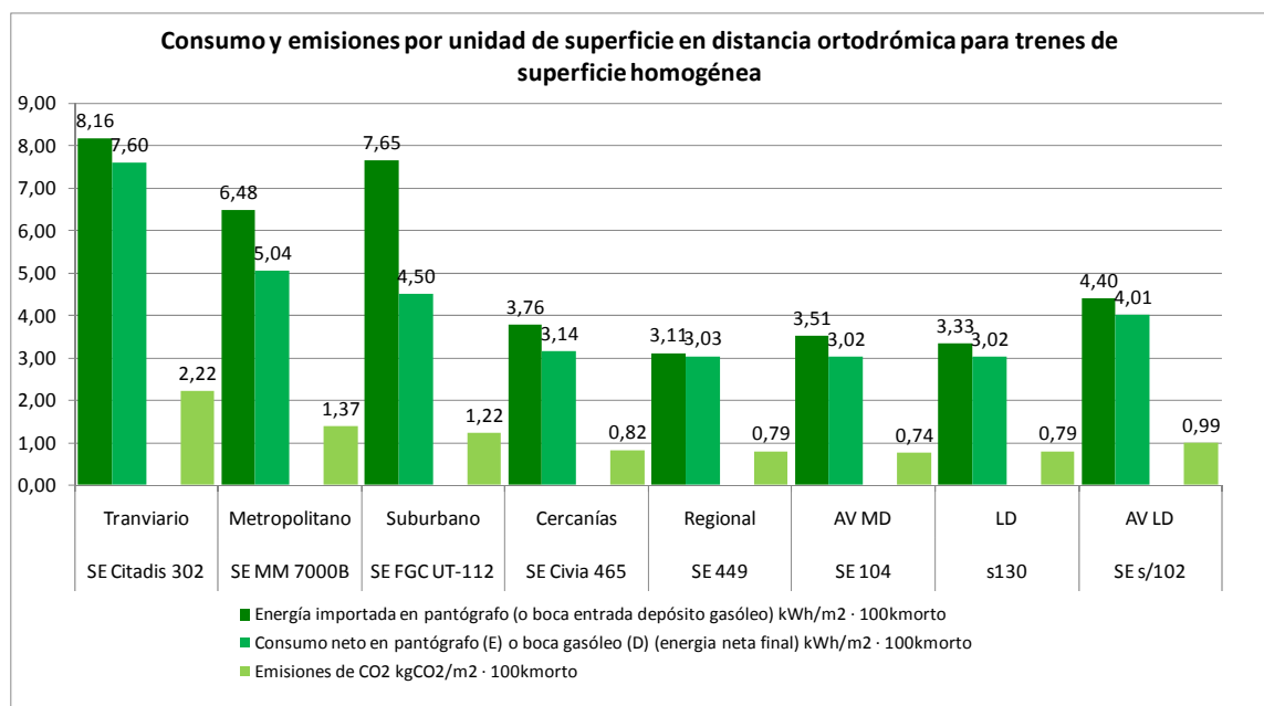
Figura 34. Consumo y emisiones por unidad de superficie y kilómetro ortodrómico
