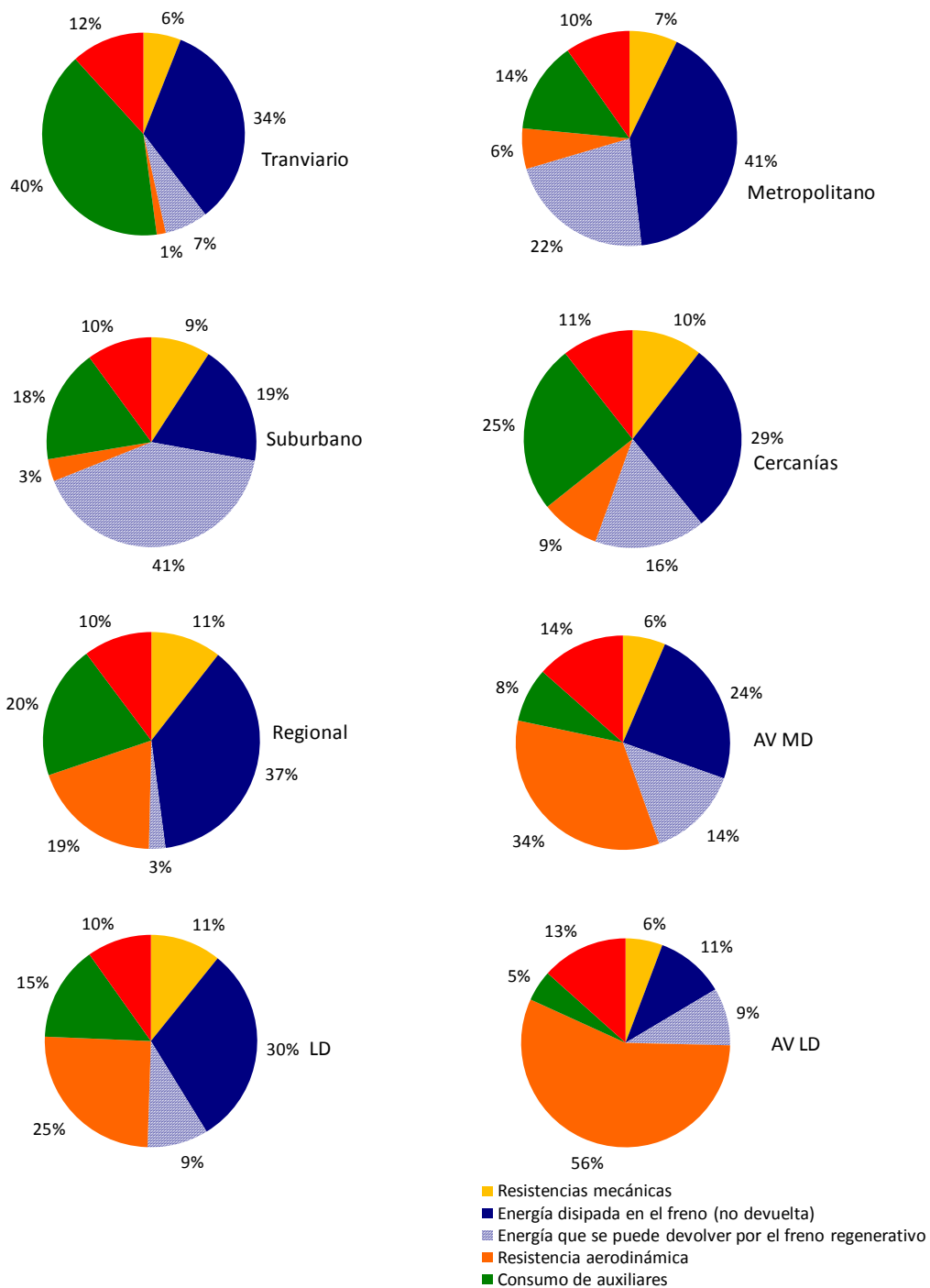
Figura 35. Peso de cada componente del consumo de energía
