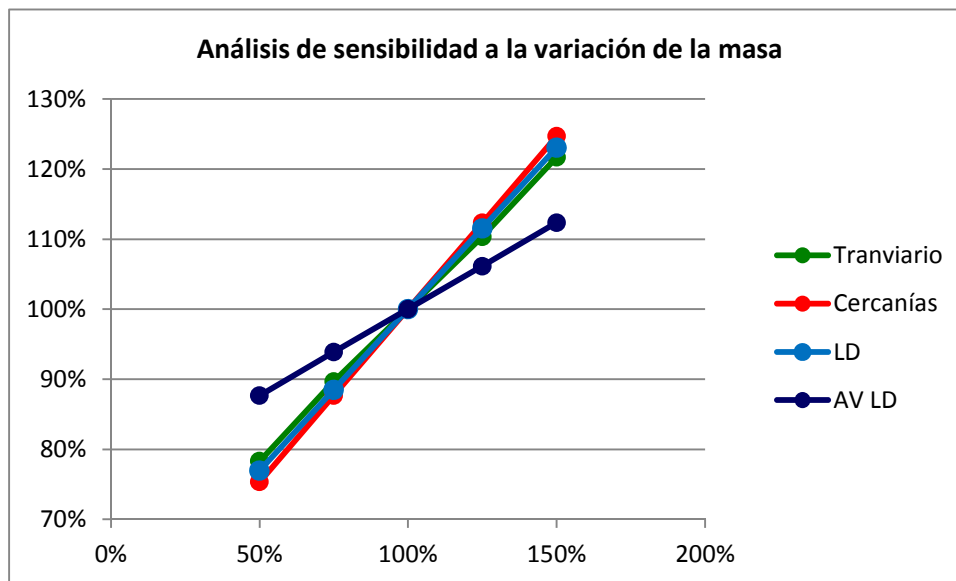
Figura 36. Sensibilidad a la variación de la masa
