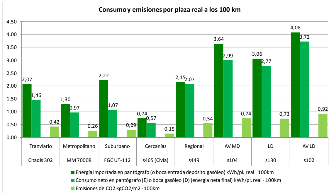
Figura 31. Consumo y emisiones por plaza real y kilómetro
